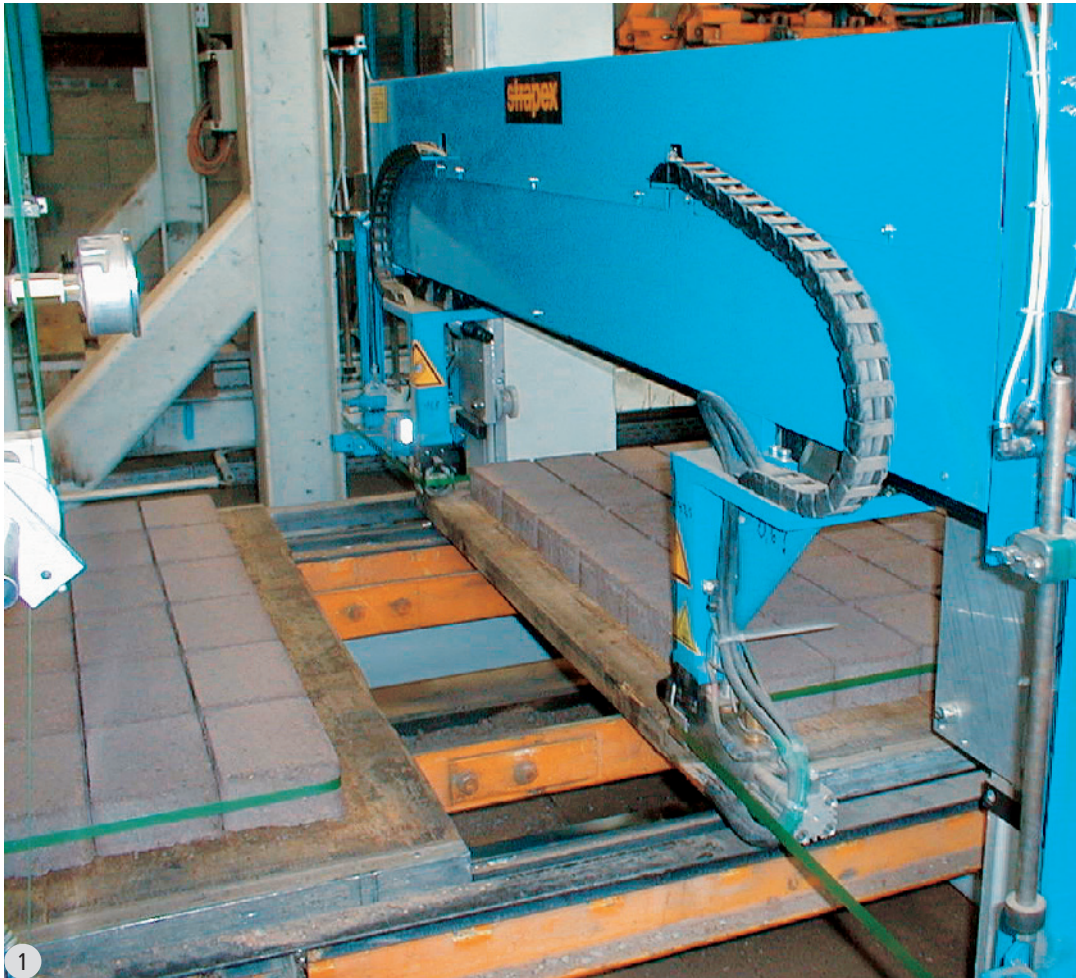
Strapex Endsealer – le système de cerclage
